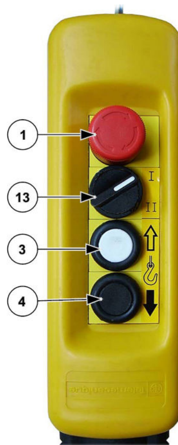
Abb. 48: Bodensteuerung/Handsteuerung (Stellung I)
