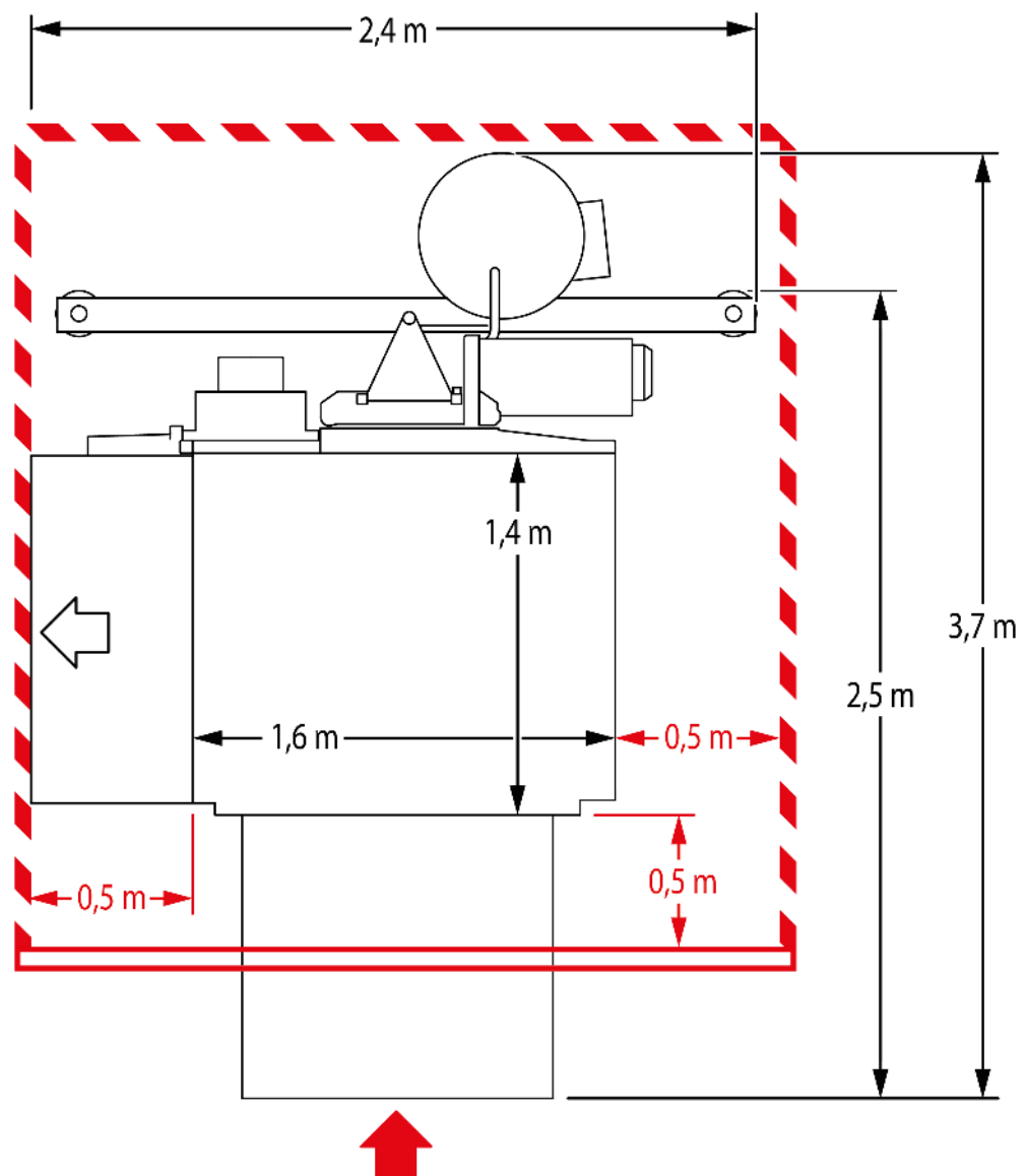
Abb. 7: Platzbedarf Bühne B
