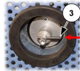
Abb. 25: Türschloss verriegelt
