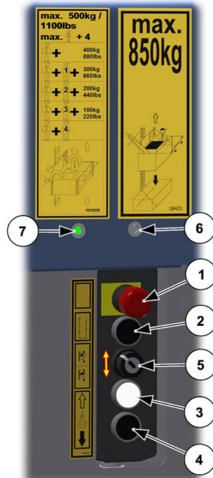
Abb. 53: Bühnensteuerung aktivieren
