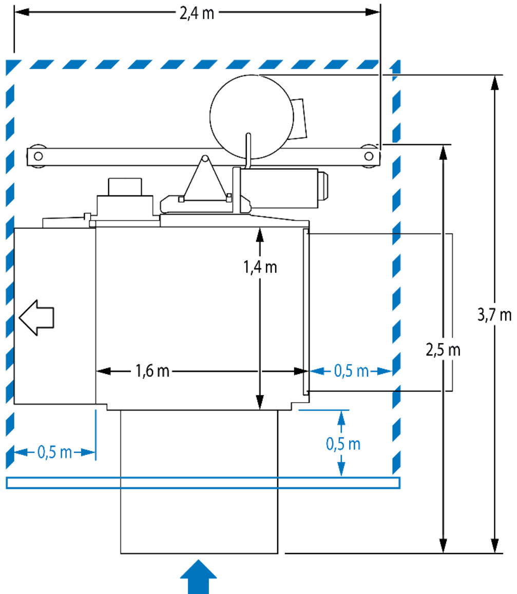
Abb. 10: Platzbedarf Bühne C Beladung C-seitig
