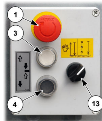
Abb. 51: Bodensteuerung für Umweh rung (AUTOMATIK)
