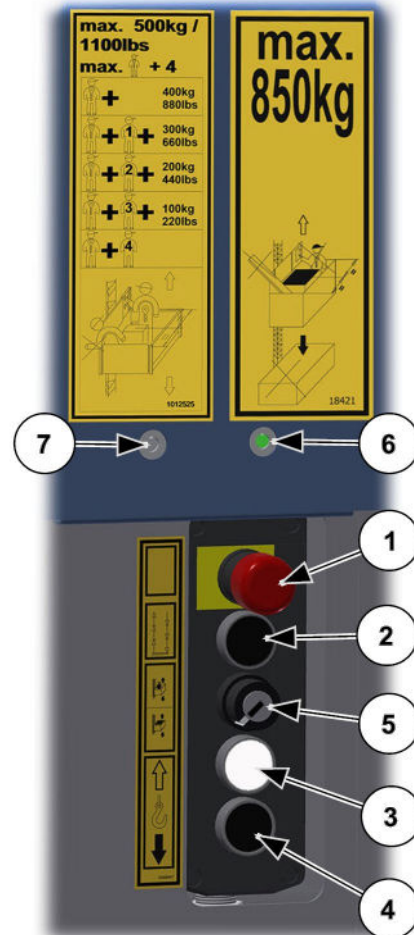
Abb. 47: Außensteuerung aktivieren
