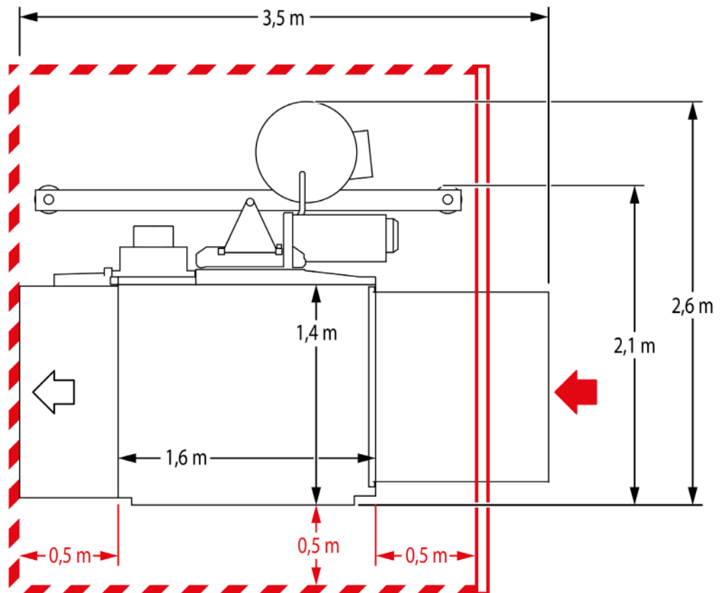
Abb. 5: Platzbedarf Bühne A
