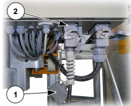
Abb. 74: Blindstecker Fangprobensteuerung
