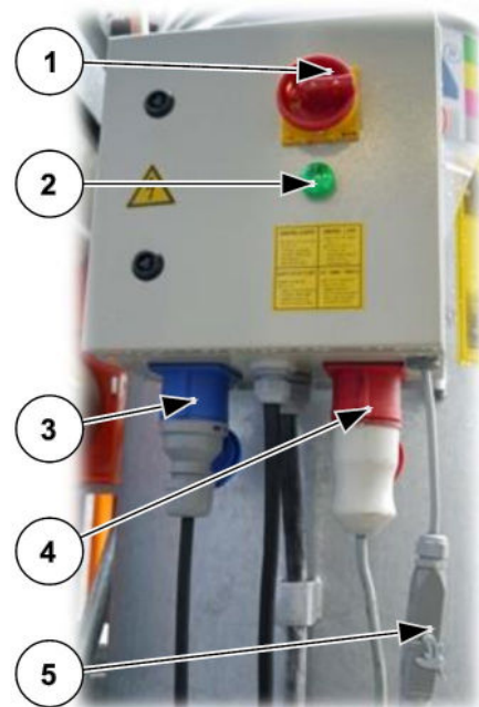
Abb. 13: Schaltkasten Bodenstation
