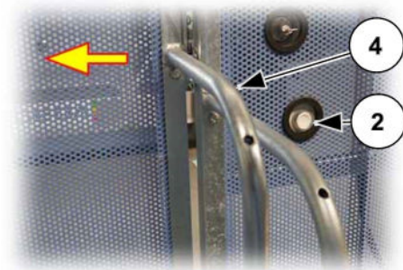
Abb. 20: Schiebetür öffnen
