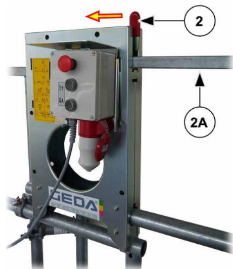
Abb. 43: Etagensicherungstür "Comfort" öffnen/schließen
