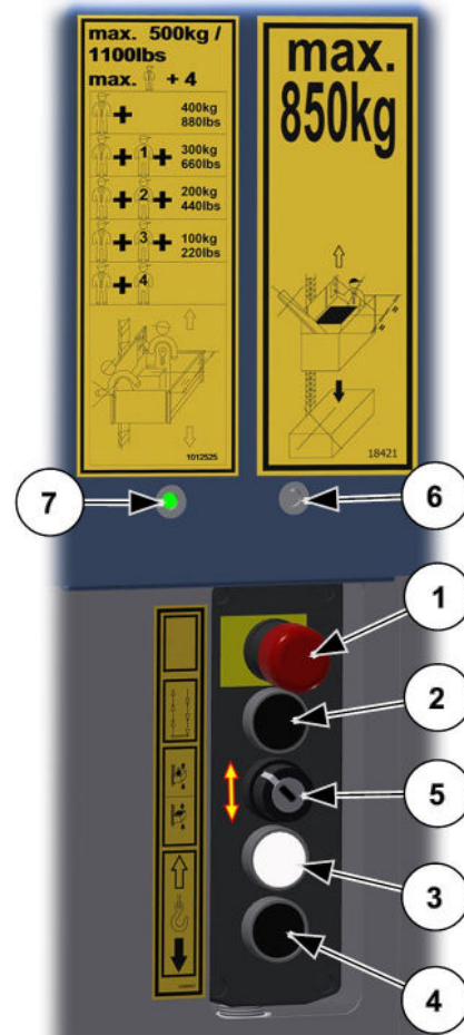
Abb. 77: Steuerung Bühne / Bedienung Transportbühne
