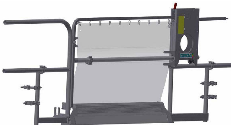
Abb. 41: Etagensicherungstür "Comfort" geschlossen (Plane)
