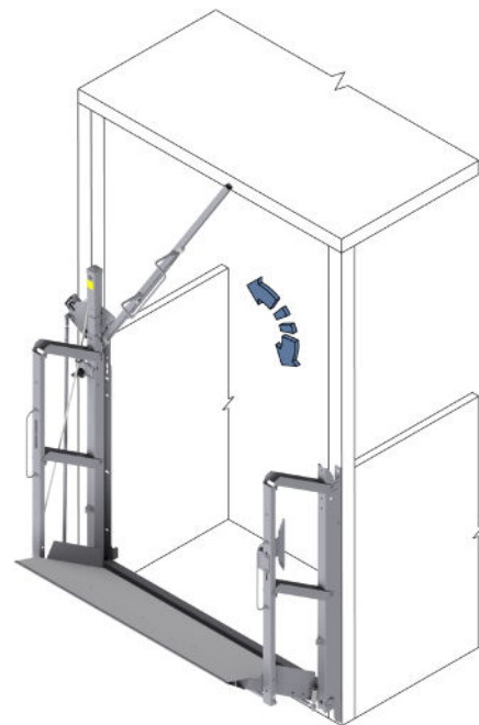
Abb. 33: Schranke mit mechanischer Verriegelung schließen
