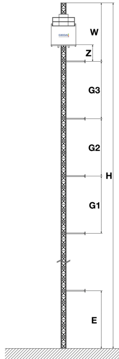
Abb. 3: Verankerung schematisch
