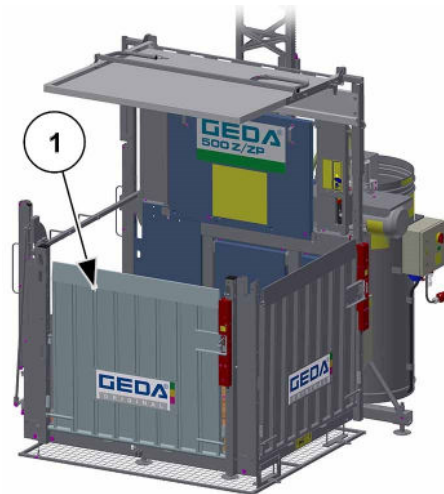
Abb. 27: Bühne mit frontseitiger Rampe
