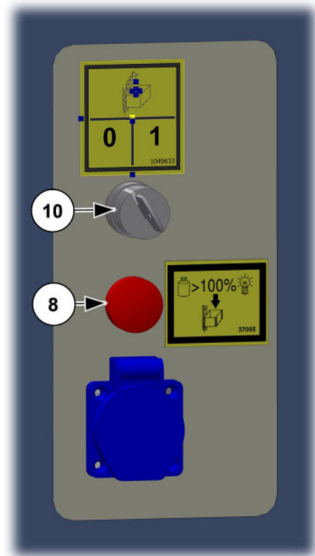
Abb. 73: Überlastanzeige
