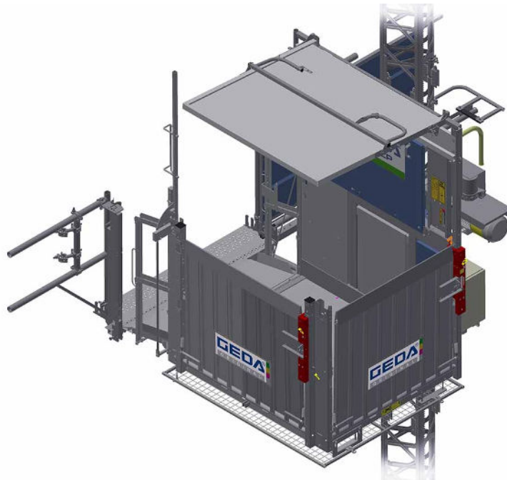
Abb. 30: Bühnenzugang Etage
