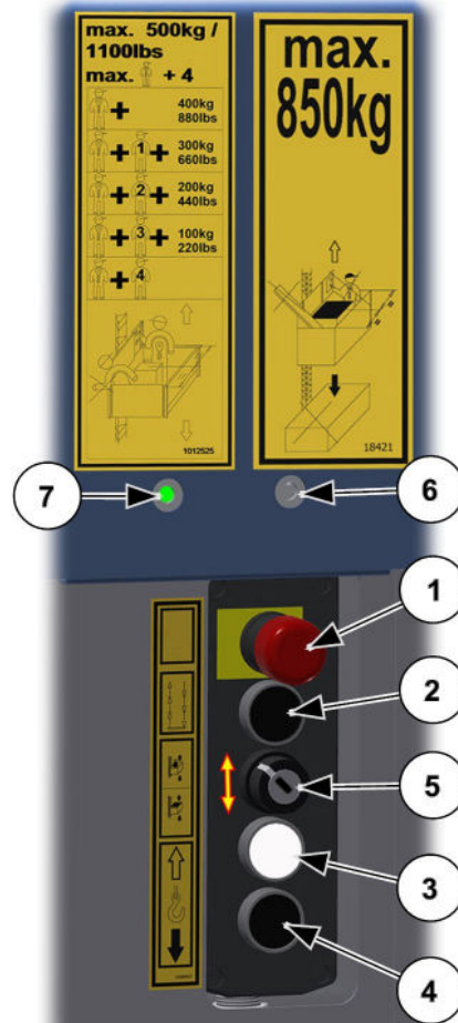
Abb. 55: Bühnensteuerung zur Montage
