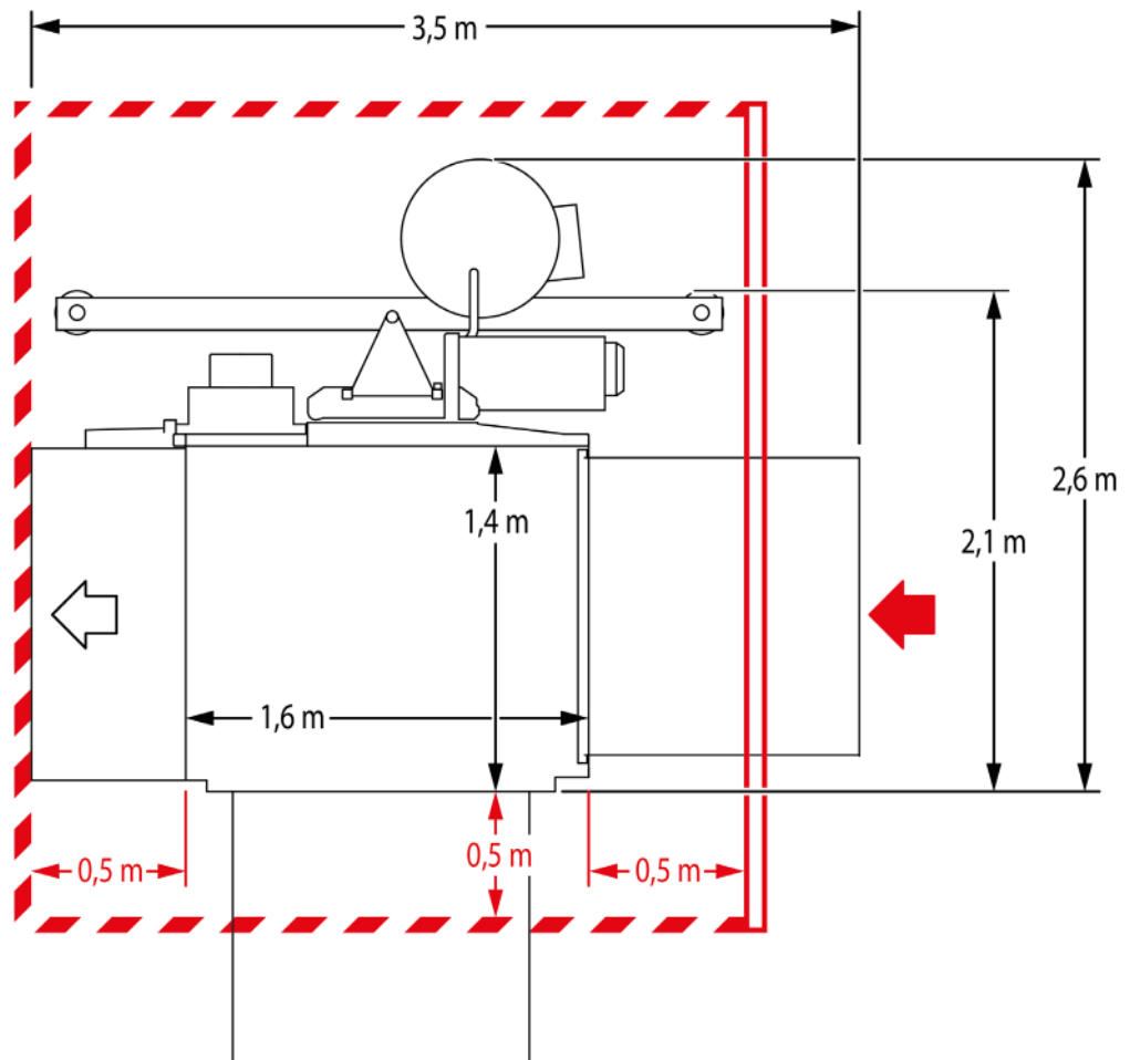
Abb. 9: Platzbedarf Bühne C Beladung B-seitig
