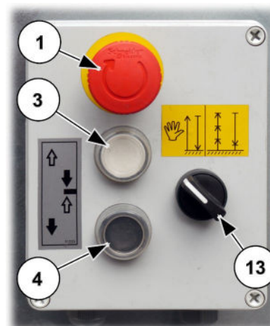
Abb. 49: Bodensteuerung für Umweh rung (HAND)
