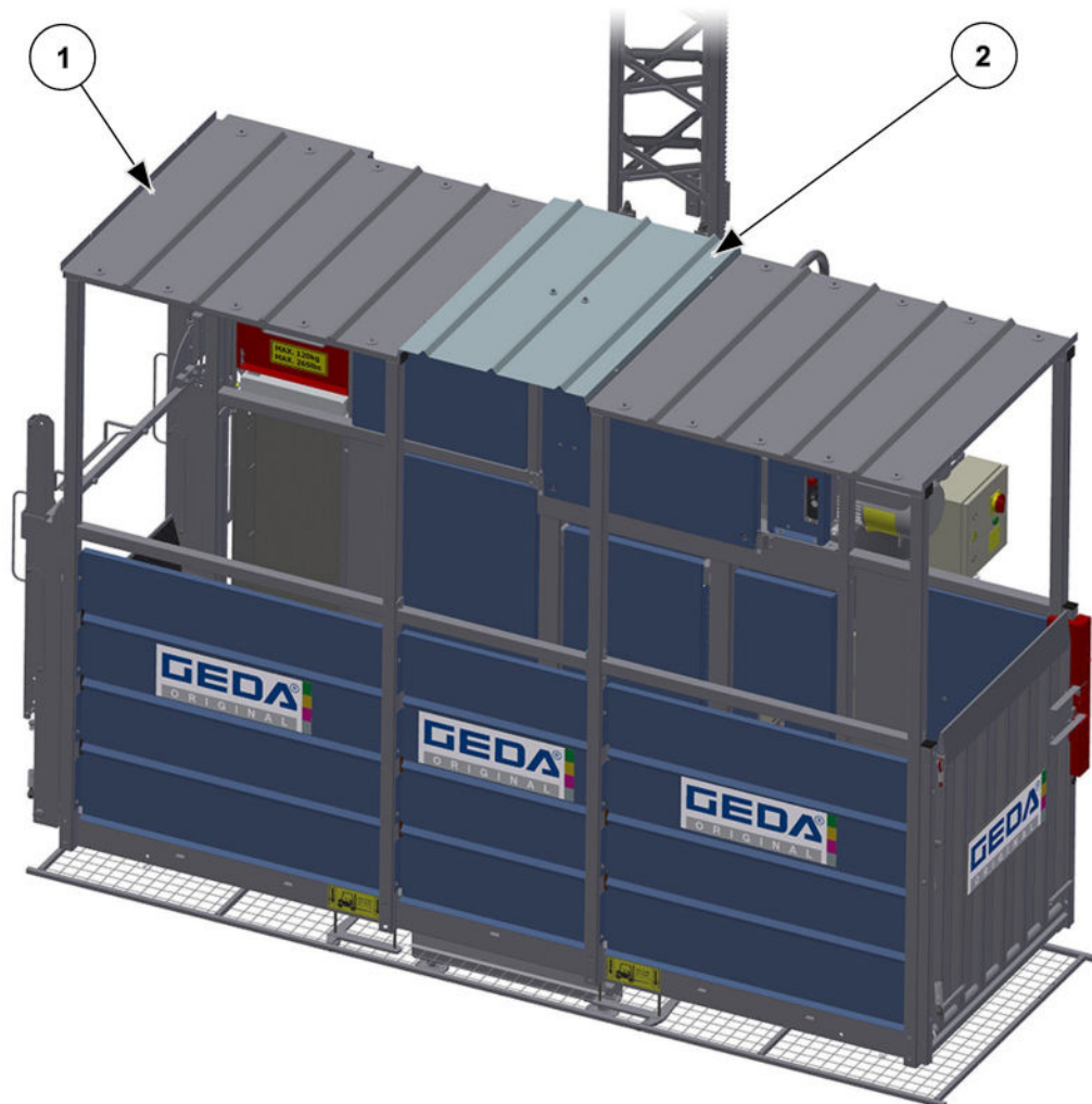
Abb. 60: Dach mit einer Montageöffnung
