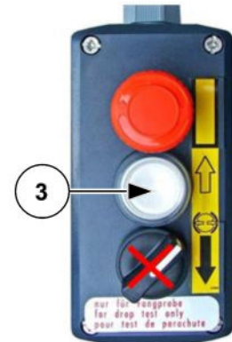
Abb. 72: Bedienung Fangprobensteuerung
