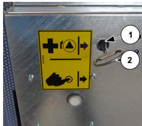
Abb. 23: Schiebetür Notentriegelung von außen
