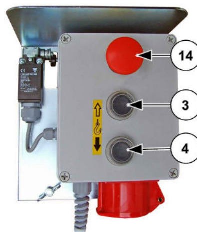
Abb. 52: Elektromodul für Etagensicherungstür
