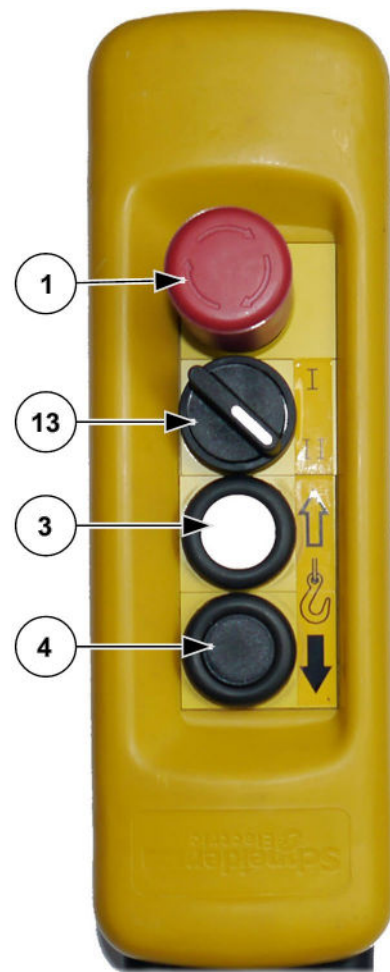
Abb. 50: Bodensteuerung/Handsteuerung (Stellung II)
