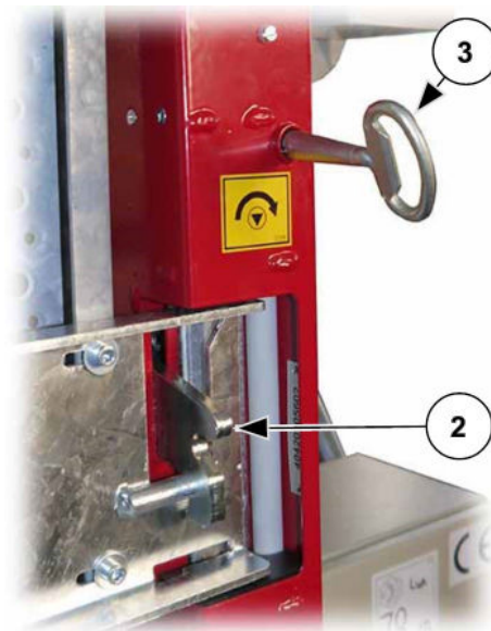
Abb. 29: Notentriegelung Rampe / Beladetür
