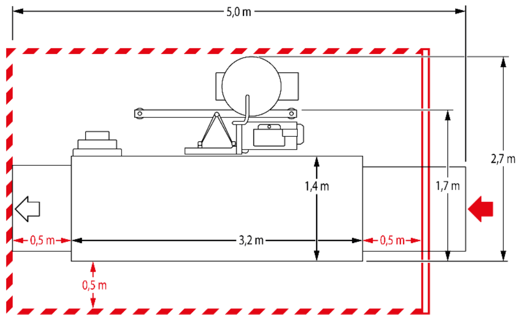
Abb. 12: Platzbedarf Bühne SL
