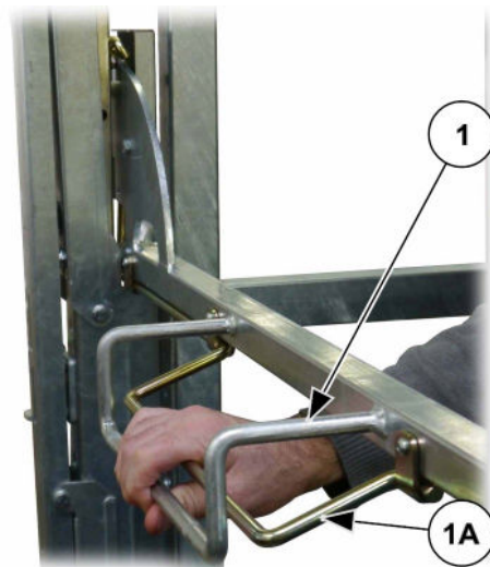
Abb. 32: Schranke mit mechanischer Verriegelung öffnen
