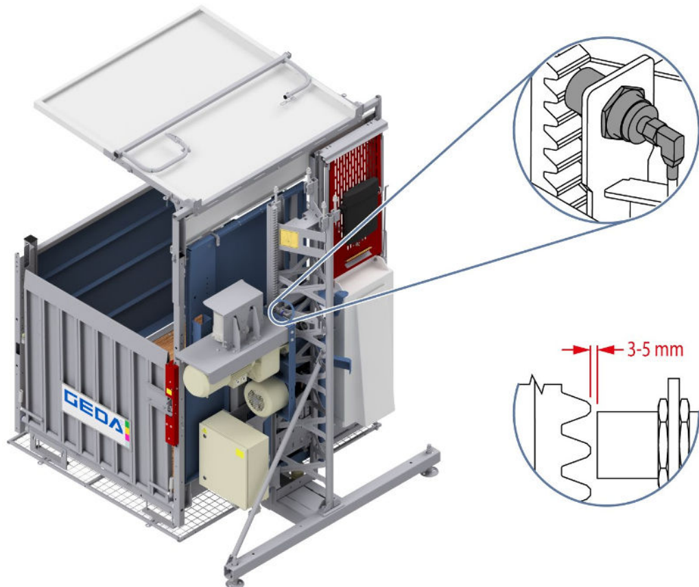
Abb. 62: Überfahr- und Kabelschutz
