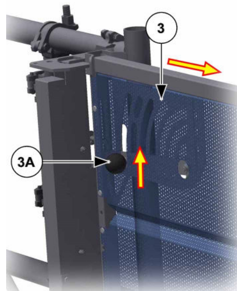
Abb. 45: Etagensicherungstür "VARIO" öffnen/schließen
