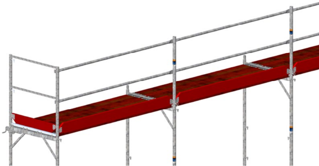
Bild 46: Vollständiger Seitenschutz
