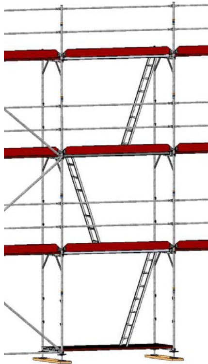
Bild 49: Innenliegender Leitergang
