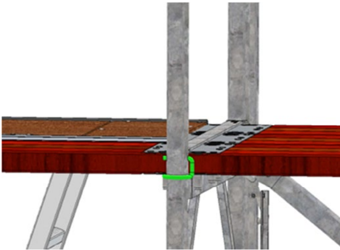
Bild 32: Eingesteckter Fallstecker.
