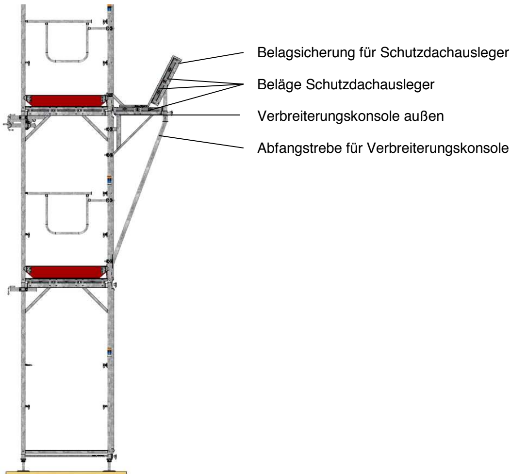
Bild 58: Schutzdach
