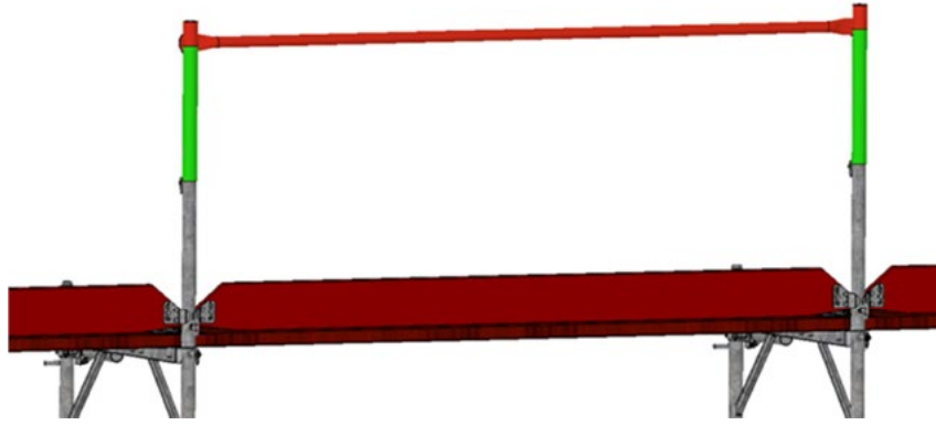
Bild 24: Empfohlene Anschlagpunkte beim oberen Gerüstabschluss
