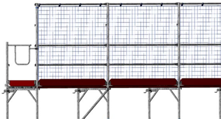
Bild 60: Schutzwand auf Vertikalrahmen.
