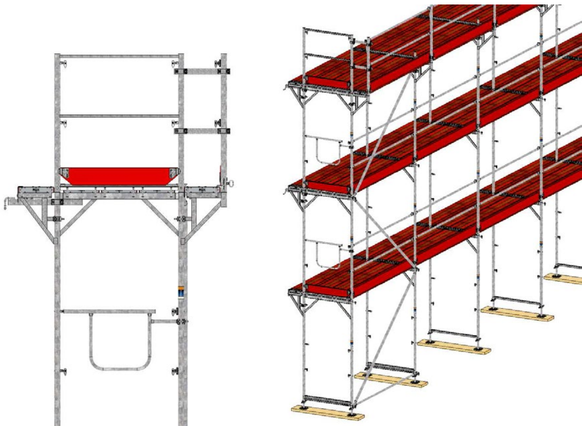
Bild 51: Gerüst mit einbohliger Verbreiterungskonsolen außen
