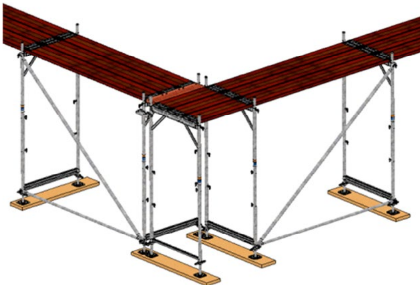
Bild 19: Eckausbildung mit drei Vertikalrahmen
