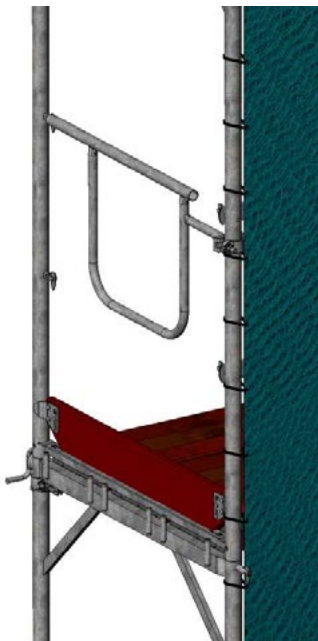
Bild 63: Bekleidung mit Netzen
