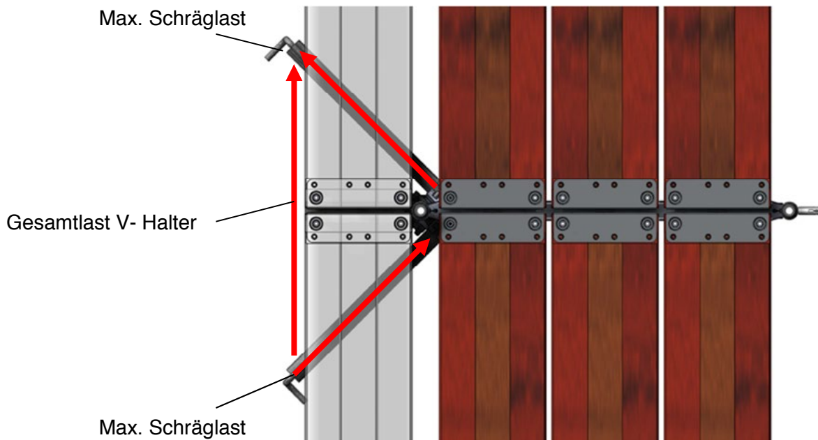
Bild 40: Kräfte am V-Halter
