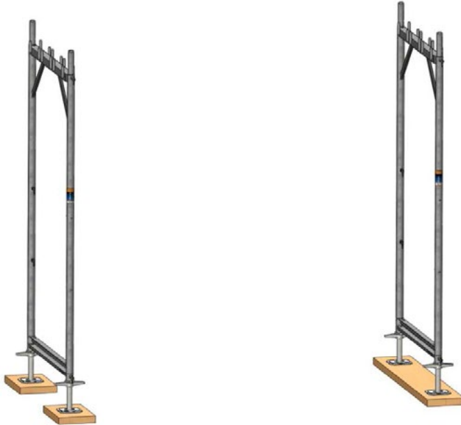
Bild 6: Aufbau des ersten Gerüstfeldes: Vertikalrahmen
