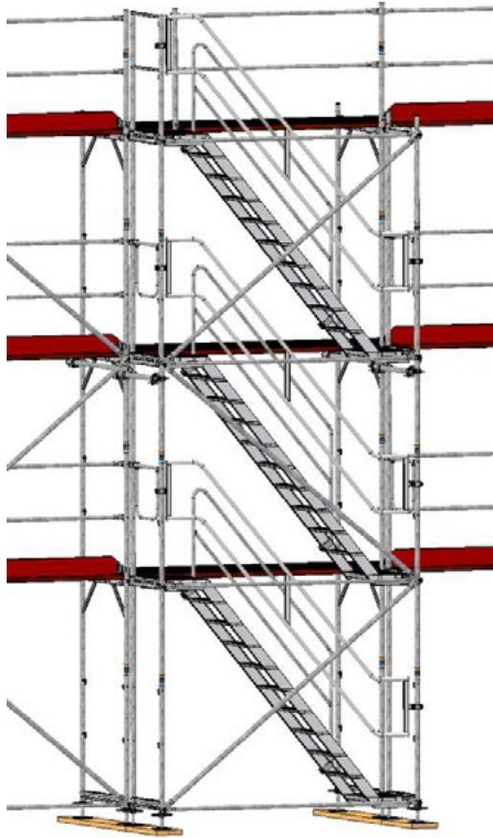
Bild 47: Vorgestellter Treppenaufstieg
