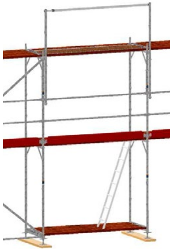
Bild 34: Montiertes MSG nur im Aufstiegsfeld.
