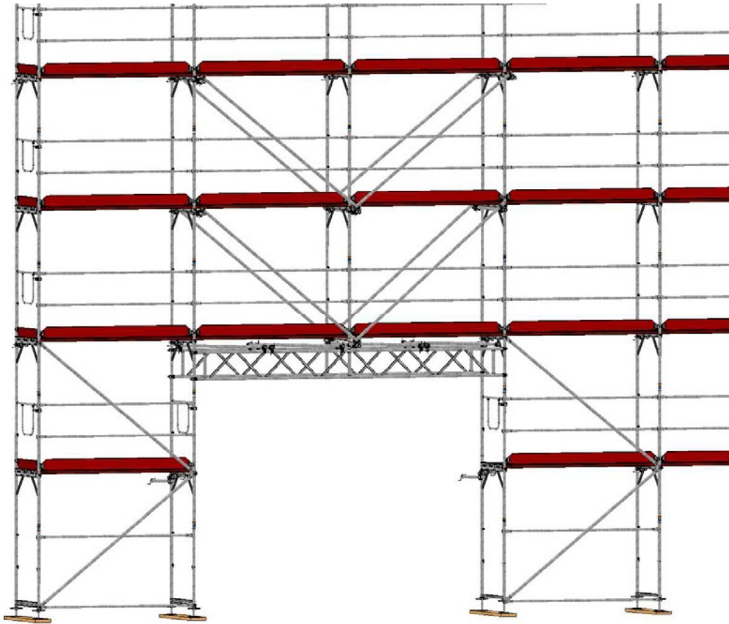
Bild 54: Überbrückung
