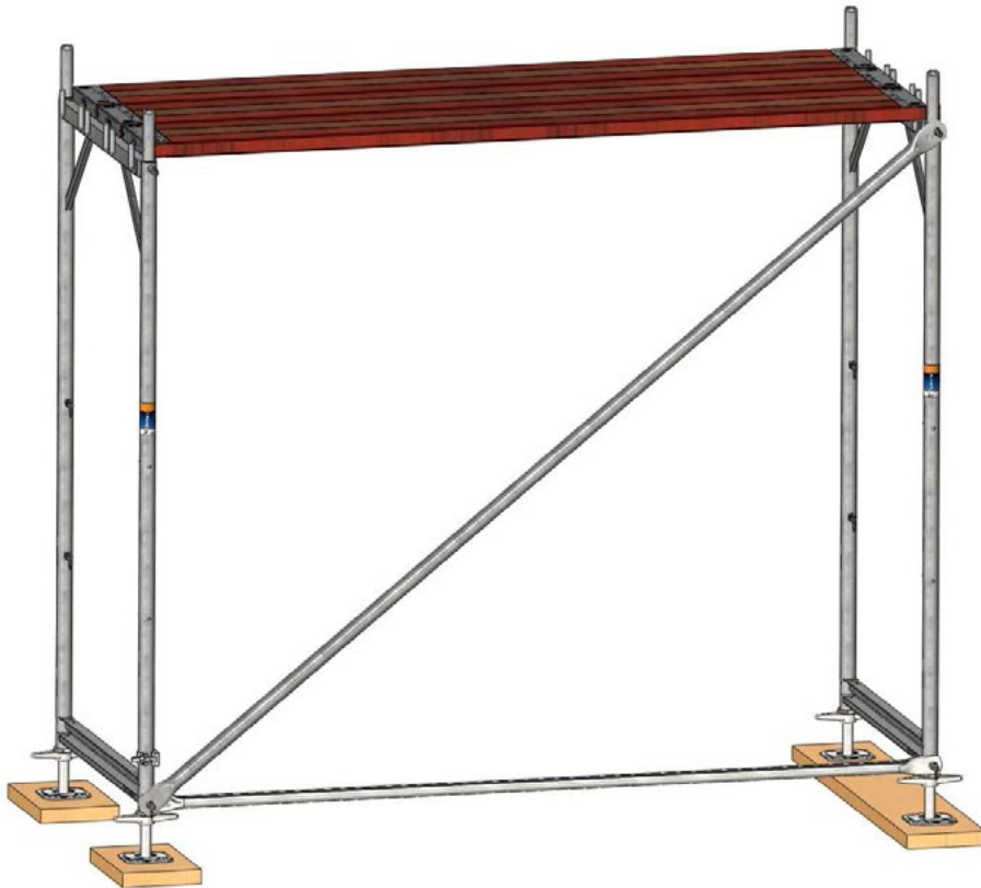
Bild 16: Fertig montiertes erstes Gerüstfeld
