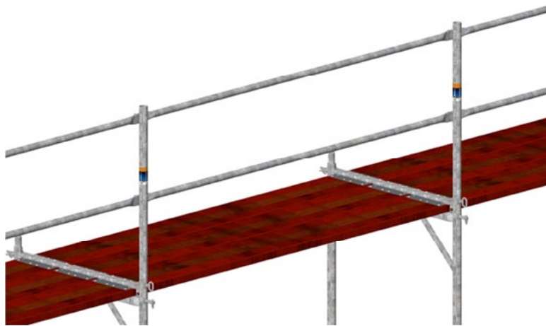
Bild 45: Oberer Abschluss mit Geländerpfosten und Belagsicherungen.
