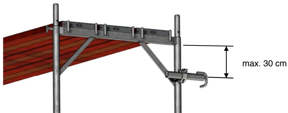
Bild 43: Verankerungen mit abweichender Ankerposition
