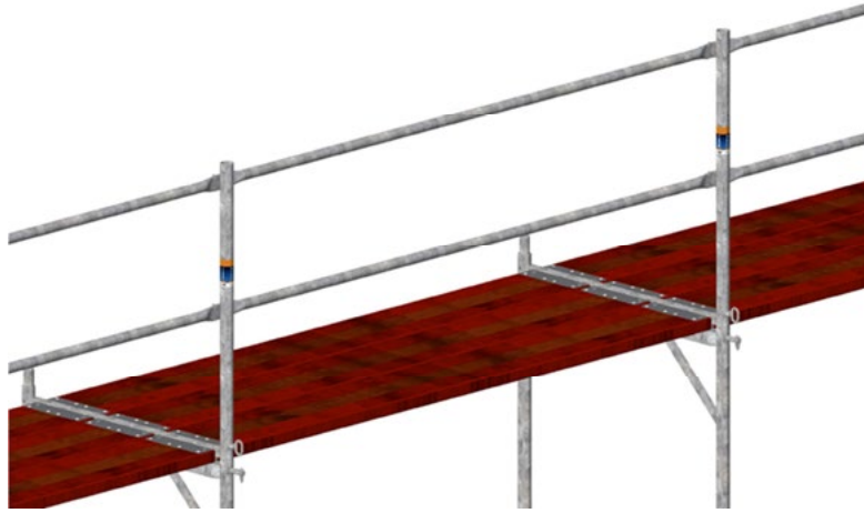
Bild 44: Oberer Abschluss mit Geländerpfosten mit Traversen.
