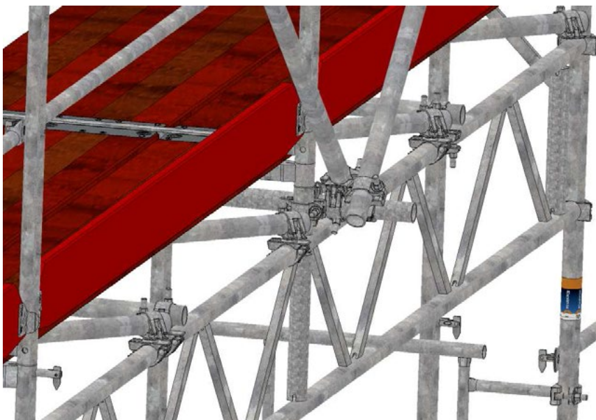
Bild 57: Anschluss der Diagonalen mit Normkupplungen
