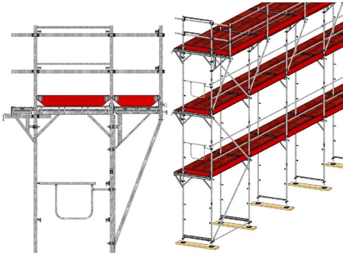
Bild 52: Gerüst mit zweibohliger Verbreiterungskonsolen außen und Abfangstrebe
