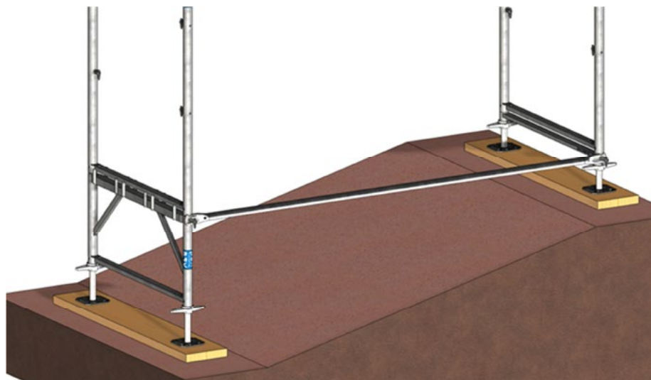
Bild 5: Ausgleichsrahmen mit 0,50 m bzw. 1,00 m Höhe.
