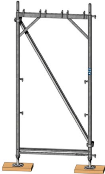
Bild 14: Vertikalrahmen mit Querdiagonale.
