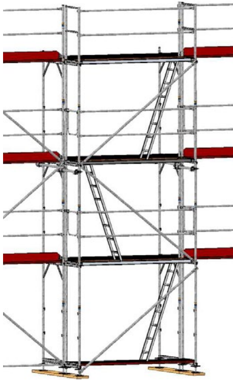
Bild 48: Vorgestellter Leiteraufstieg.
