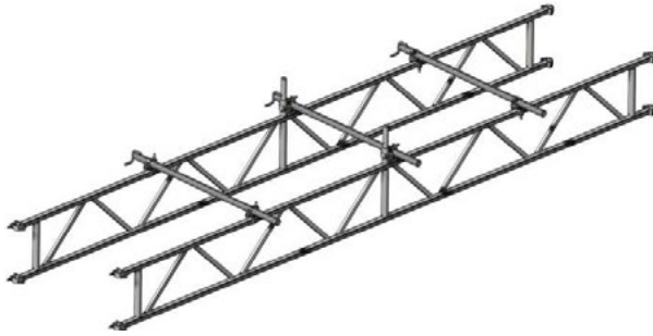
Bild 55: Horizontalaussteifung mit Verankerung
