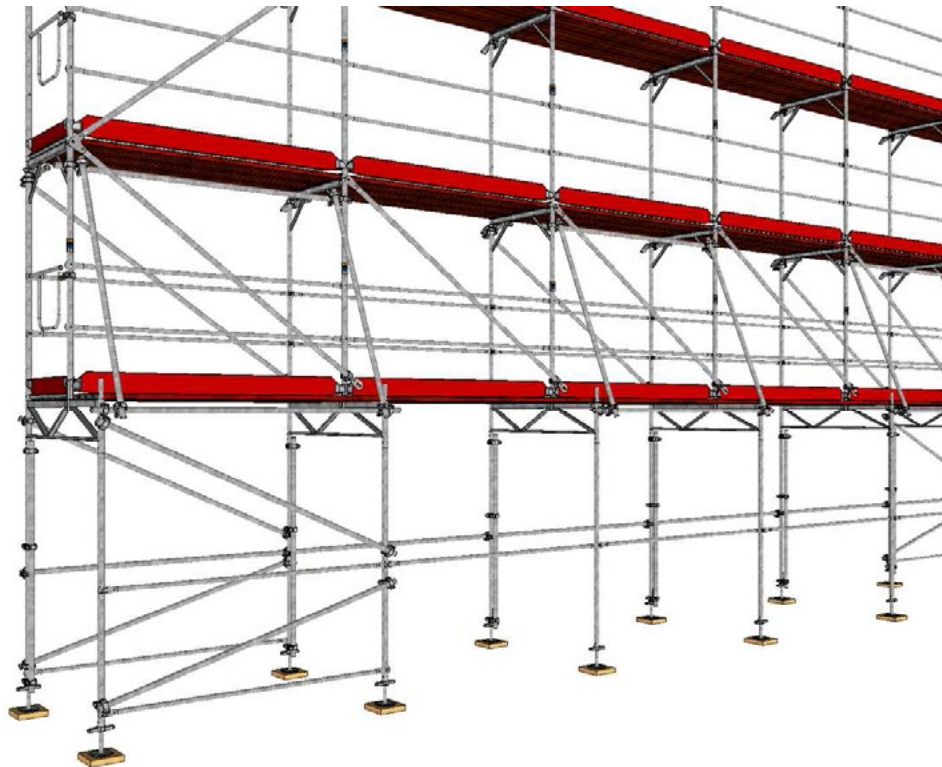
Bild 53: Durchgangsrahmen
