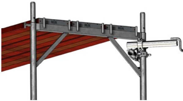
Bild 38: V-Halter, Grundkonfiguration
