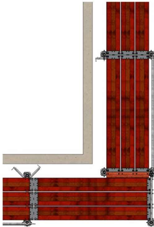
Bild 41: Verankerungen im Eckbereich, Ausführung mit zwei Vertikalrahmen
