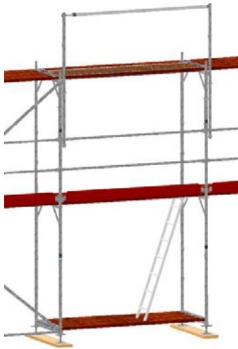
Bild 28: Einhängen des zweiten MSG-Pfosten.
